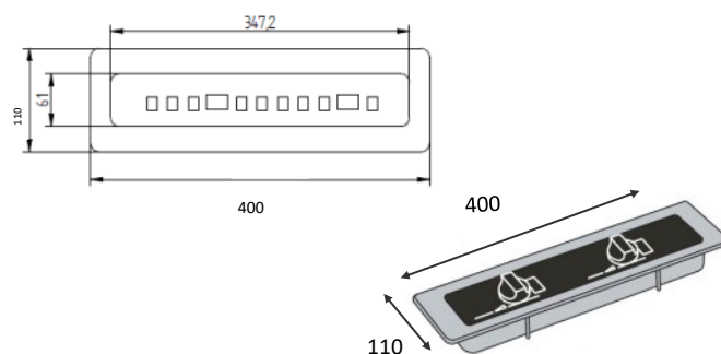
Dimensions découpe: 367x72mm
